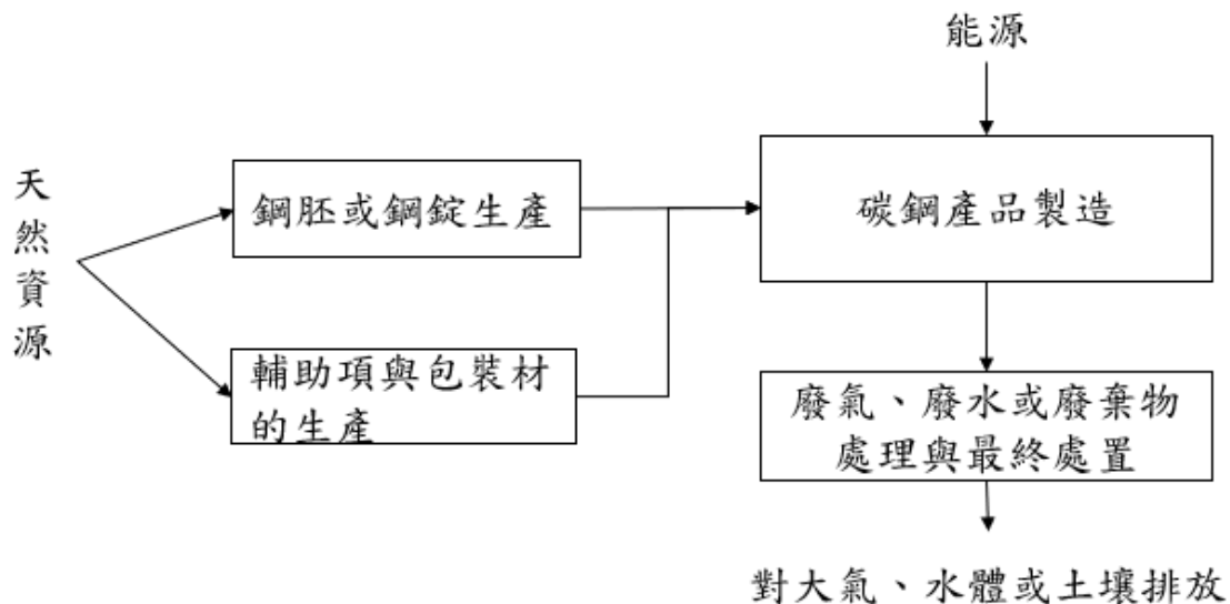
圖3、碳鋼產品類別的系統圖
