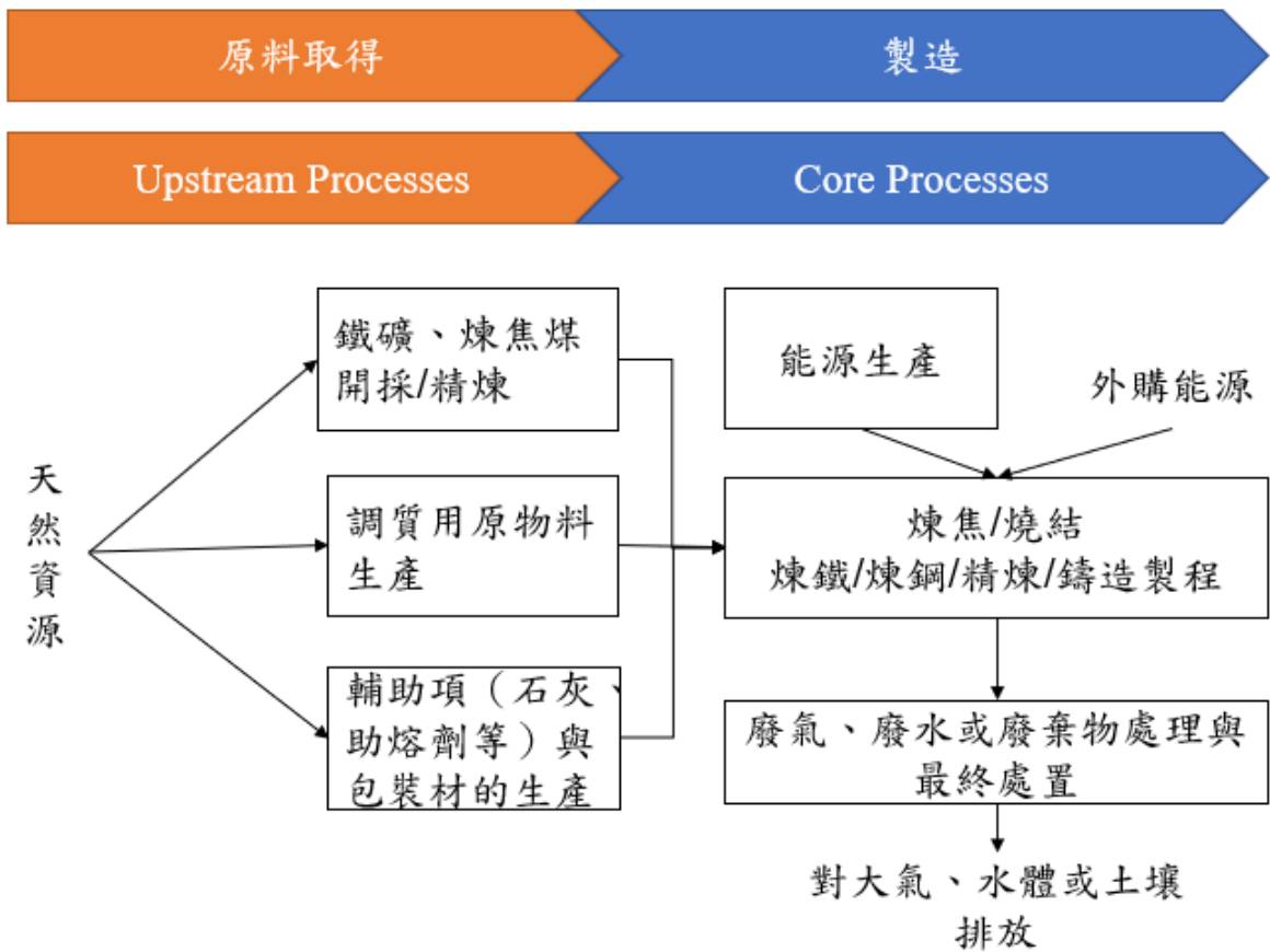
圖1、高爐 (blast furnace ,BF) 與轉爐 (basic-oxygen-furnace ,BOF) 生產碳鋼的系統圖
