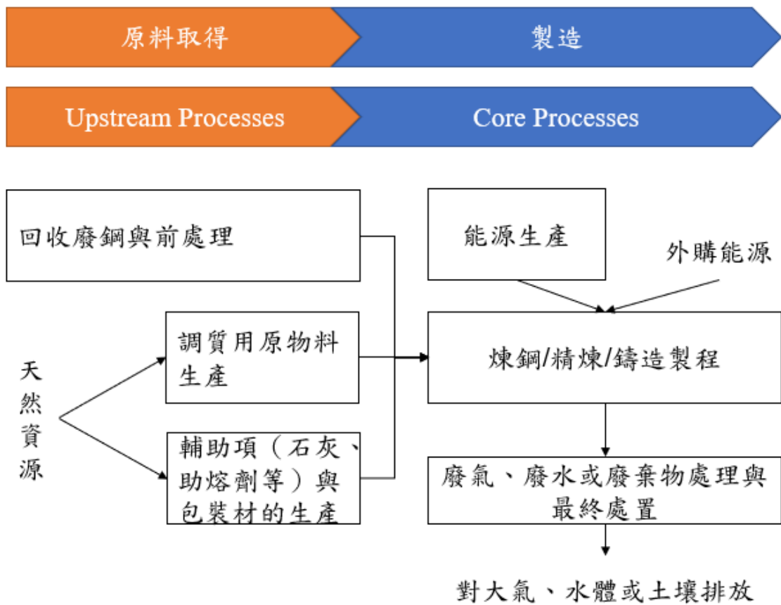
圖2、電弧爐 (electric arc furnace ,EAF) 生產碳鋼系統圖
